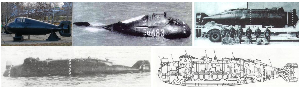
Överst t.v. och i mitten den sovjetiska 2-mansfarkosten Triton 1. T.h. 6-mansfarkosten Triton 2. Nederst t.v. en Triton 2, som har gått upp till ytan. T.h. en Triton 2 (teckning).
