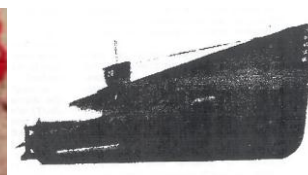
Böjd sonarbild av Oberonklassubåt. Böjd sonarbild av ubåt från Vidingefjärden 1984. COSMOS SX-506
