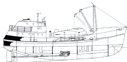
T.v. teckning av Olterra med vattenfylld sektion. I mitten och t.h. GSE:s reklam för bärare av minifarkoster.
