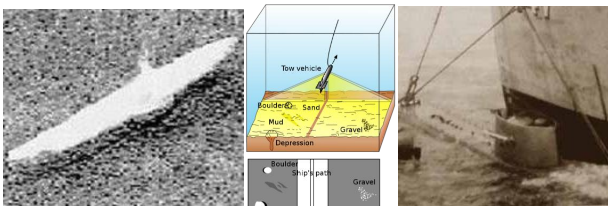
T.v. sonarbild av amerikanskt ubåtsvrak USS Wahoo . Mitten, principen för en släphydrofon med ett blint område längs färdvägen. T.h. COSMOS SX 404 (16 meter) i Taiwan. Den bärs av civilt fartyg.
